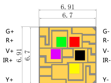
正面图
