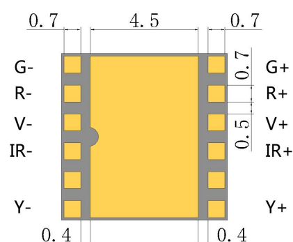
背面图
